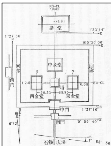
図25 飛鳥寺伽藍配置図
