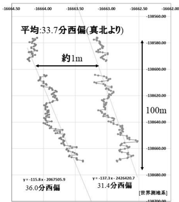
図44 恭仁京・右京中軸線下の溝の方位
