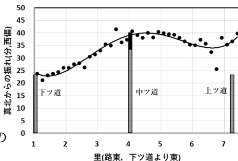
図33 南北方向の条里制地割の方位
