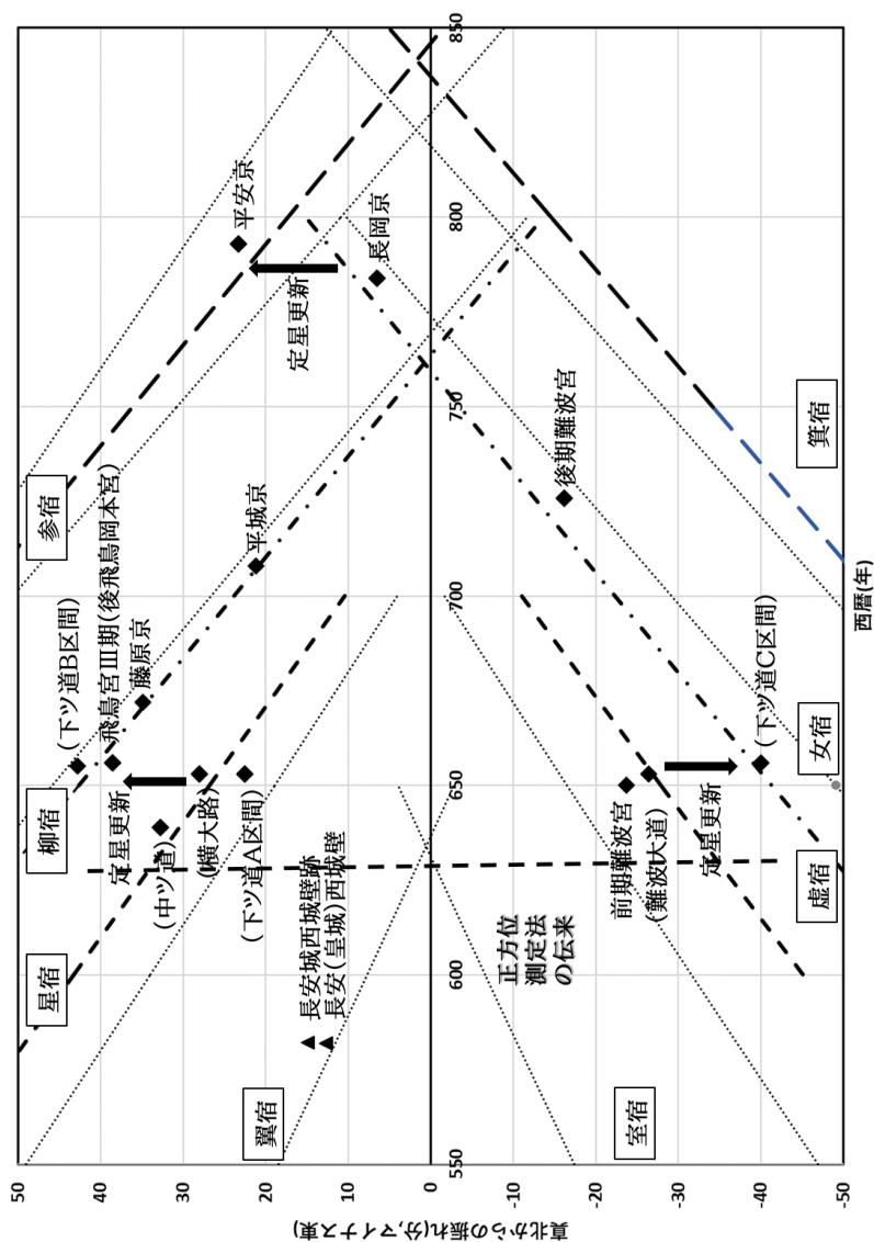
図 22 北極星(HR4893)と星宿距星による方位線と都城や大道遺構の方位 29)
