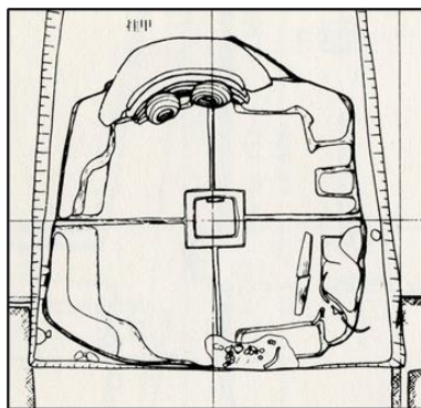
図 26 飛鳥寺塔心礎図
