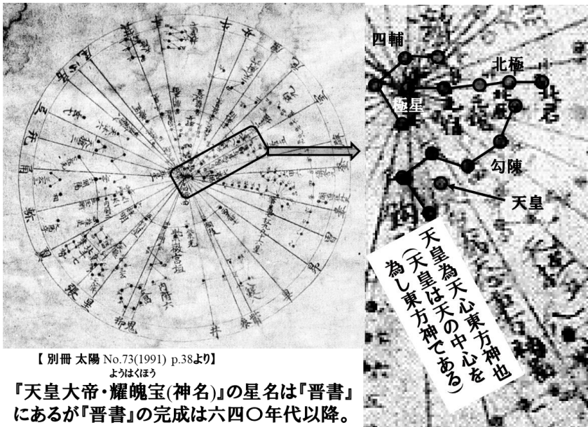
図 5 2 『格子月進図』の「天皇」星
